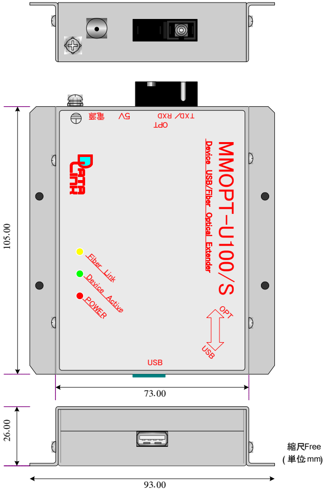
■MMOPT-U100/s 外觀図
