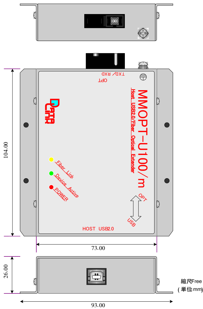
■MMOPT-U100/m 外觀図
