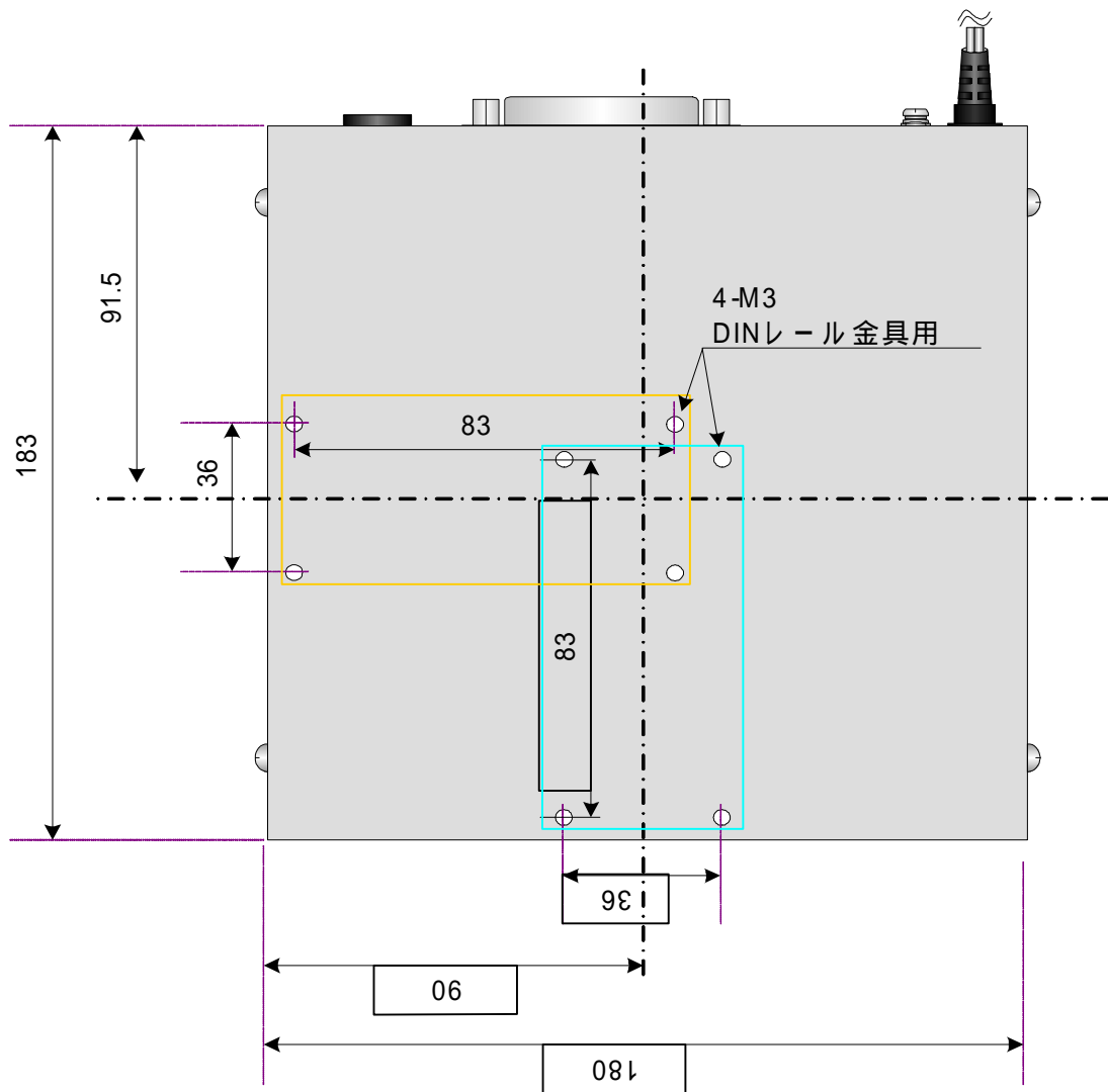
【 Enet-HDLC/ AC DINレール取付金具穴位置寸法図】
