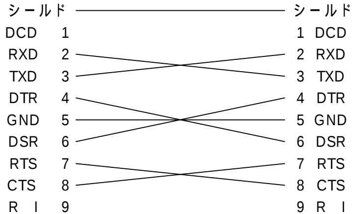
Dsub9 ピンメス - Dsub9 ピンメス クロスカбель結線図
